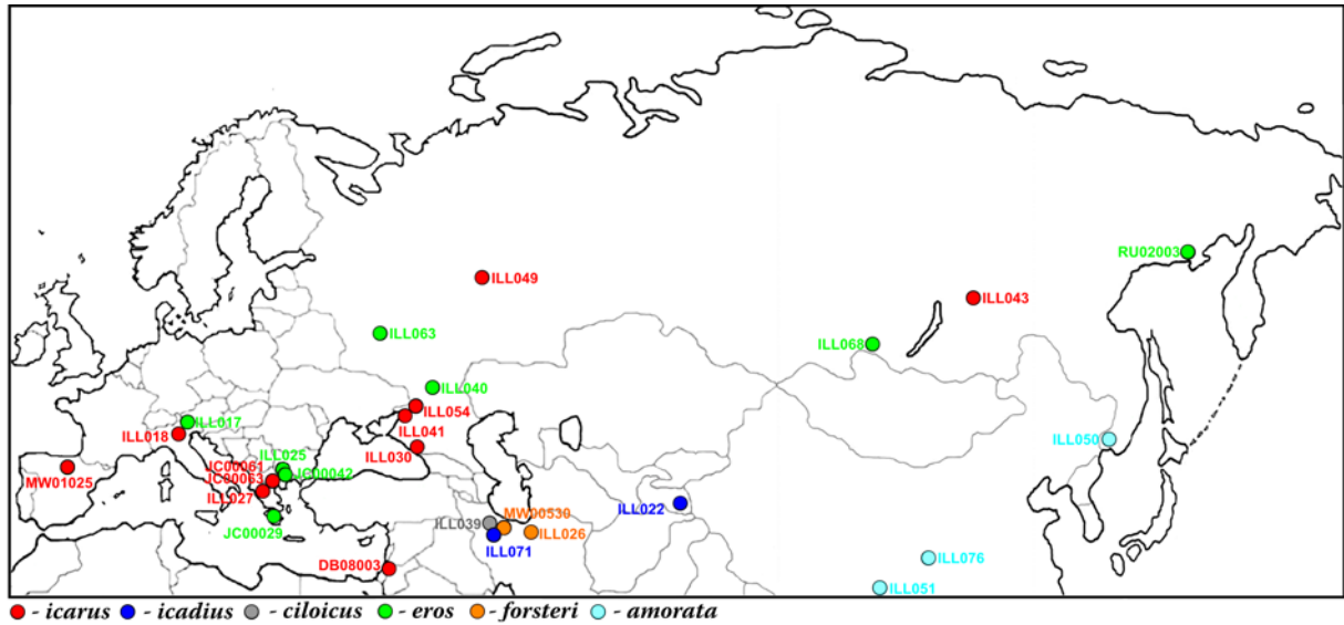
Рис. 1. Локализация изученных экземпляров Polyommatus (см. Приложение 1). Fig. 1. Collecting localities of examined specimens of Polyommatus (see Appendix 1).
